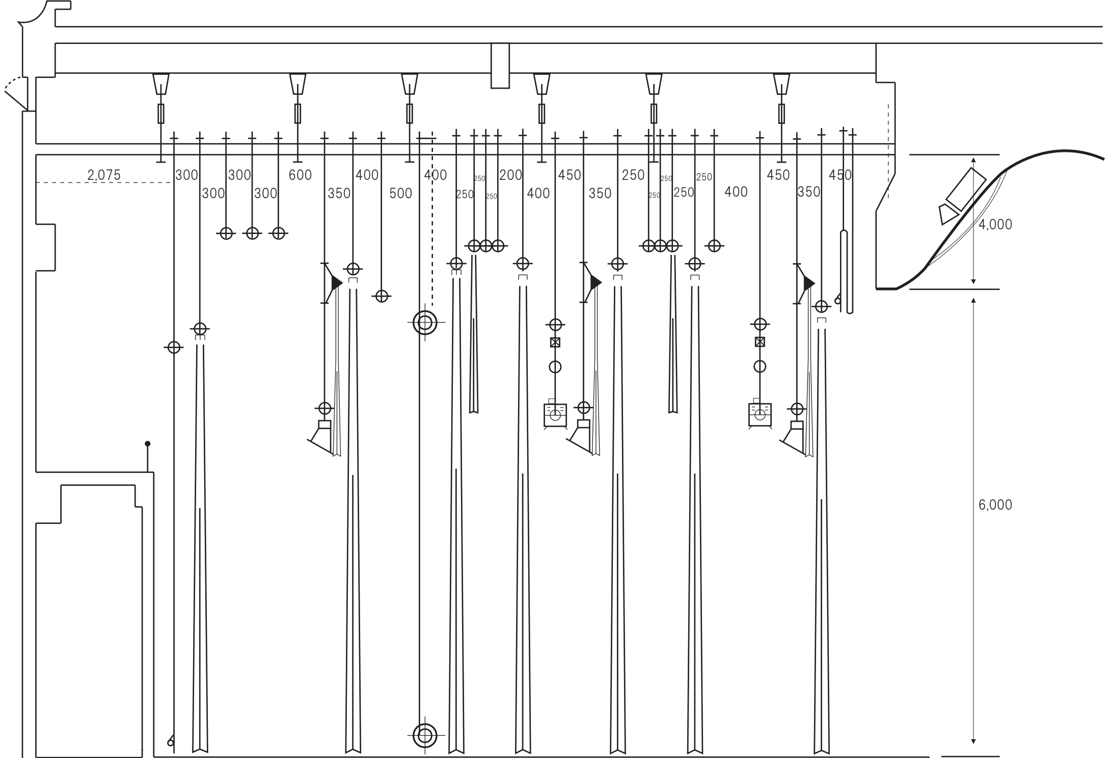
長岡市中之島文化センター 舞台 断面図
